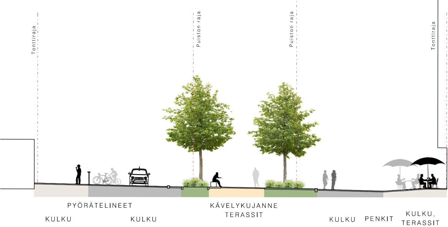
LEIKKAUS B-B 1:200
